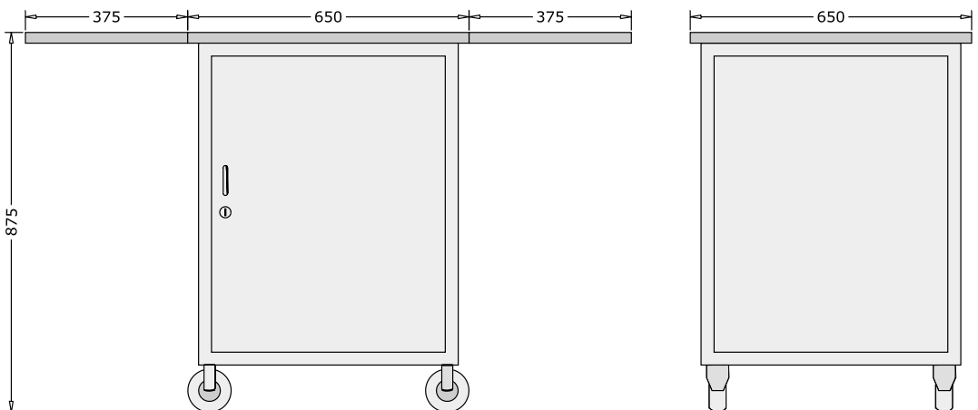
Unterschrank 'Mika de Luxe'
